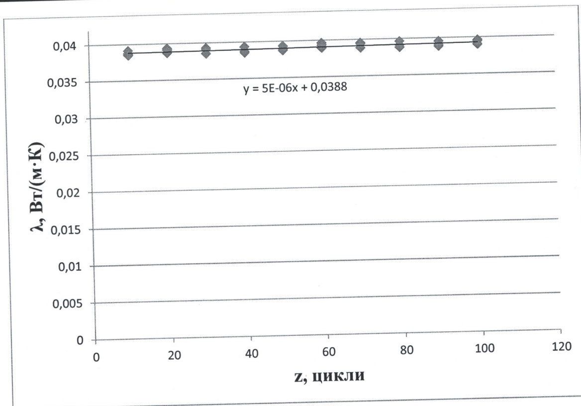
Рисунок 3 – Залежність теплопровідності від циклічних впливів
